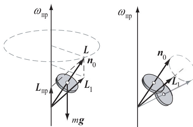
Рис. 5. Наложение нутации вокруг направления вектора L_1 на вынужденную прецессию.
